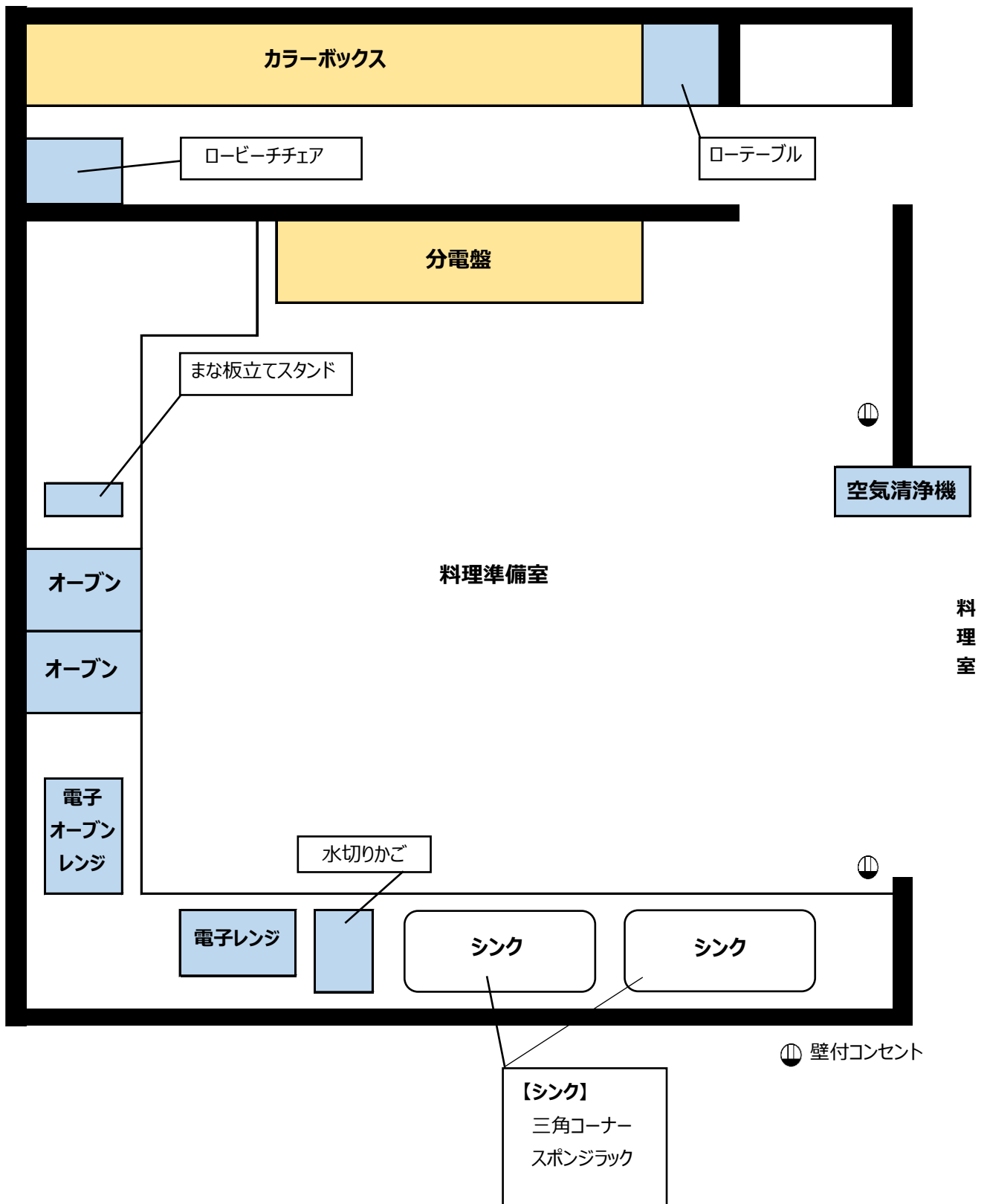
料理準備室備品配置図 1
